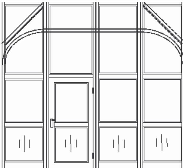
Abbildung 19: Rauchschutztüre eingebaut in Rauchschutzverglasung aus gekoppelten Seitenteilen
