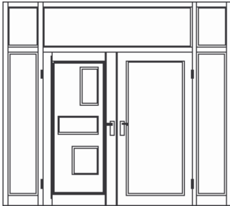
Abbildung 22: Mit Oberlicht und zwei schmalen Seitenteilen, geschoßhoch
